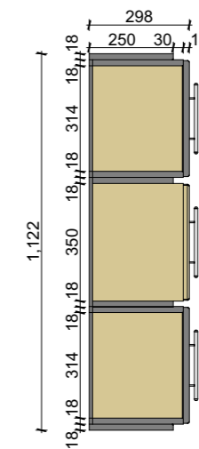
Corp S4 S 1:20
