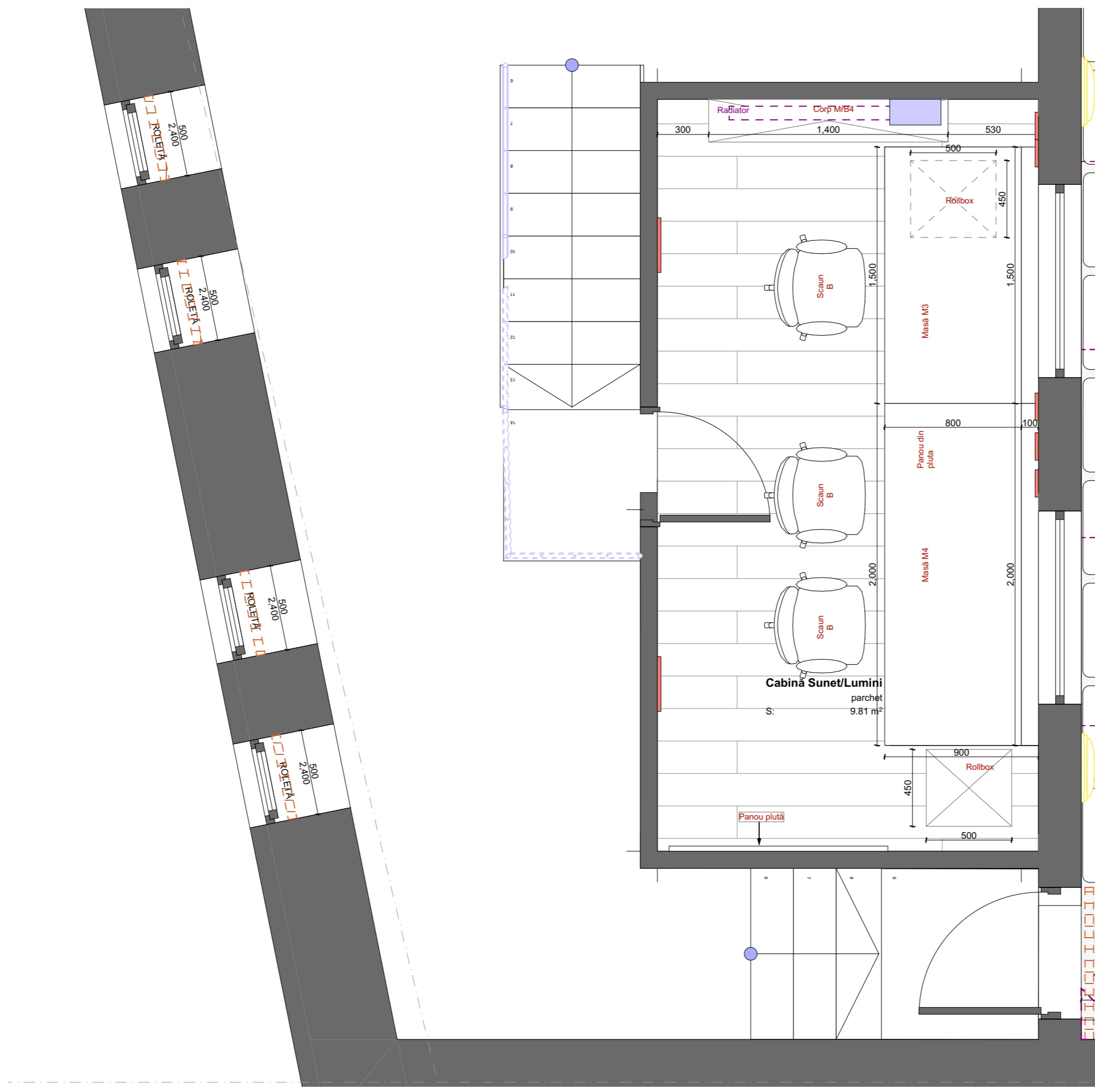
0. PLAN PARTER - COTA 3,10 1:25
